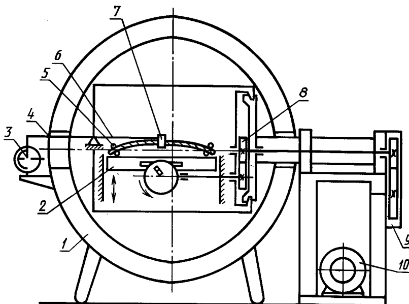
Схема стенда для определения усилия изгиба кабеля
